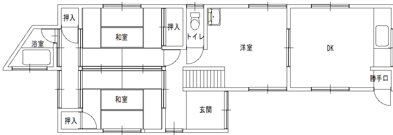
1階平面図
